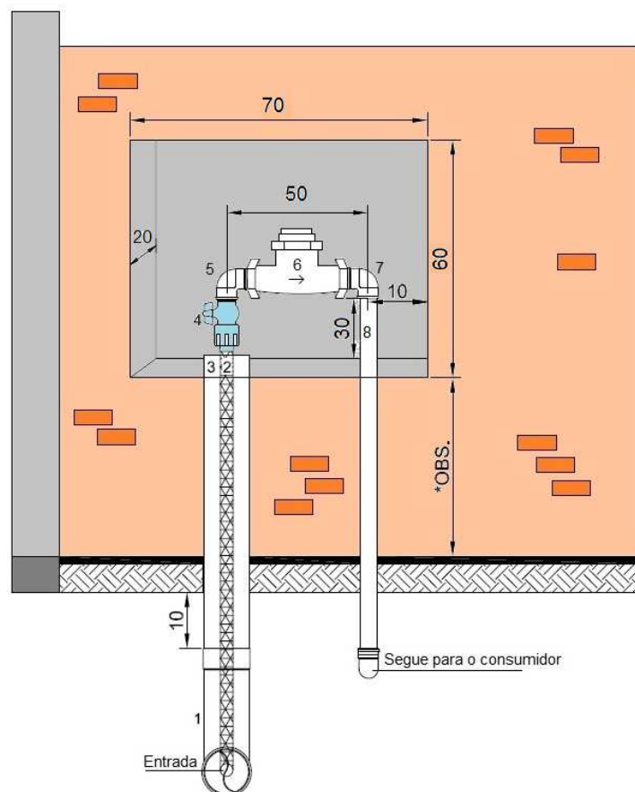
Caixa padrão para hidrômetro 1 ½"
